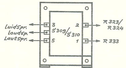
GELUIDUITGANGSTRAFO SOUND OUTPUT TRANSF. TONAUSG. ÜBERTRAGER
