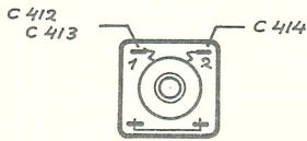
LUNOSC. SPOEL S 401 LINE OSC. COIL ZEILENOSZ. SPULE 50 156 007
