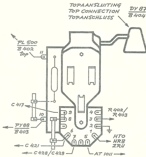
LUNUITGANGSTRAFO LINE OUTPUT TRANSF. ZEILENAUSG. ÜBERTRAGER
